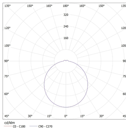
KANLUX S.A. (kat 26984) VARSO LED 24W-NW-O-SE / LDC (Polar)
